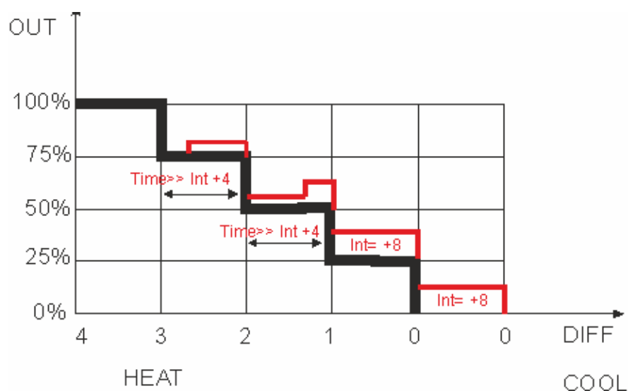
Figuur 2: voorstelling van het versnellings-/vertragsmechanisme van Qbus PID sturing
